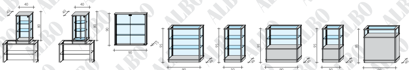
Lada przeszklona całkowicie
