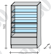
Lada witryna 100
