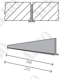
Łącznik czołowy
